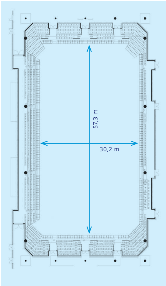
Ground dimension – Standing no tribunes Rozměr plochy – Stání bez tribun 57,3 x 30,2 m Ground dimension – Standing with tribunes Rozměr plochy – Stání s tribunami 38,9 x 20,2 m
